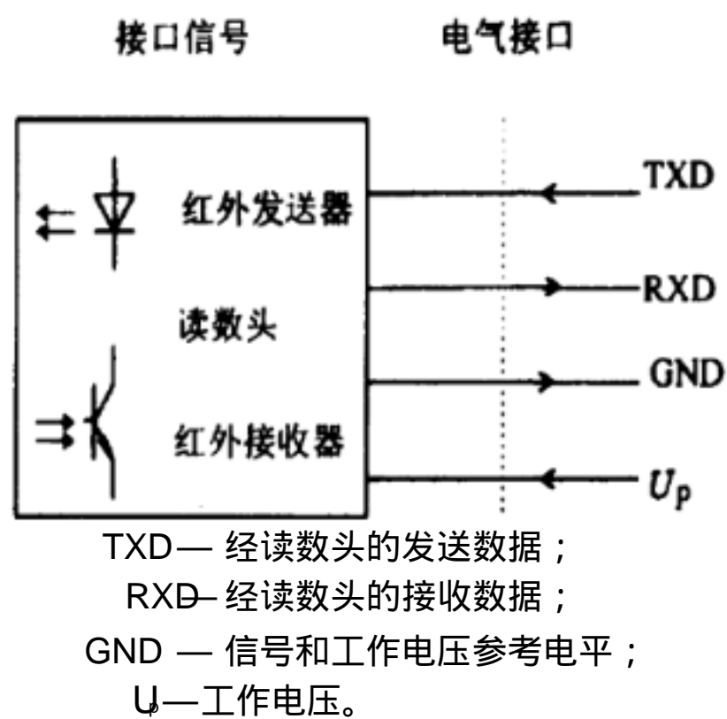
图4 读数头的电气特性
