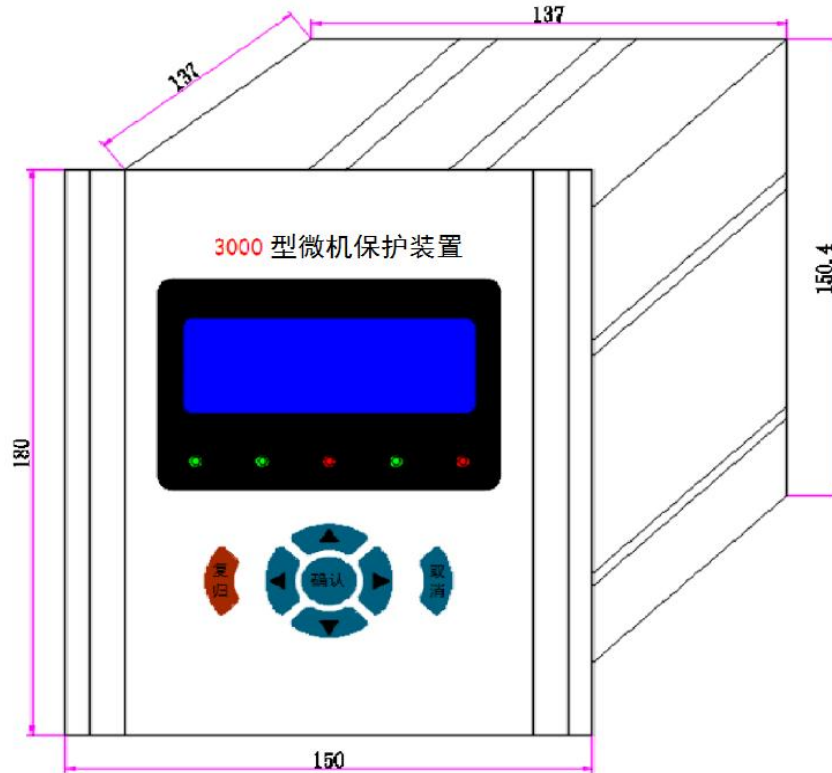
图 2-1 外形尺寸
